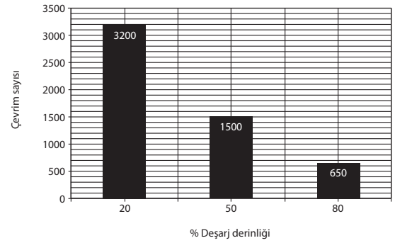
Çevrim ömrü - Deşarj derinliği +25°C
