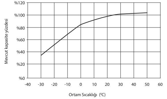
Kapasite – Ortam Sıcaklığı
